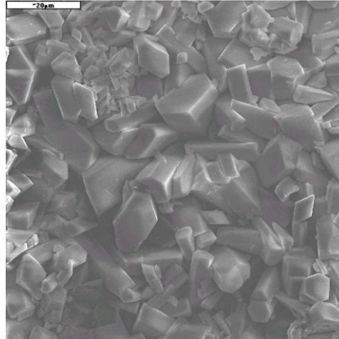
SURFACOTE MN 2, 1000x aumentos
