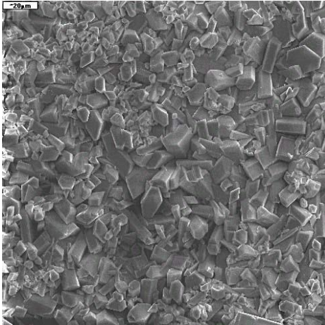
SURFACOTE MN 2, 500x aumentos
